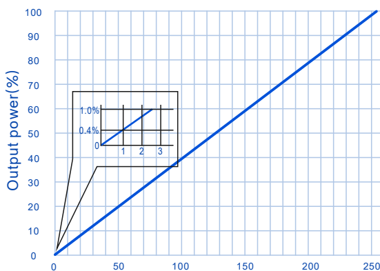
线性调光曲线: (DALI-2/DMX机型)
